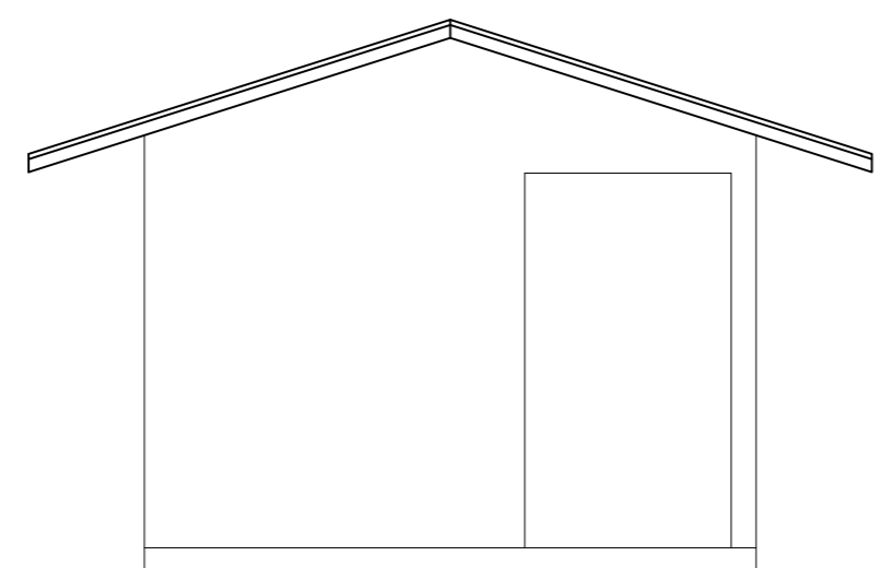
FACHADA LATERAL esc:1/50
