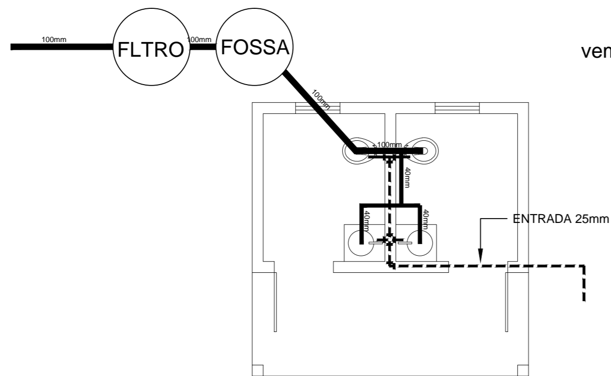
PROJETO HIDROSANITÁRIO esc:1/50
