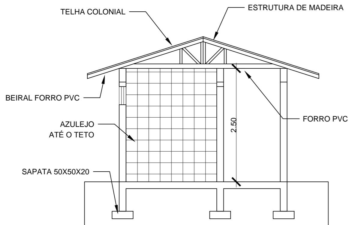
CORTE "A,B" esc:1/50
