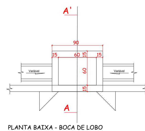
PLANTA BAIXA - BOCA DE LOBO
