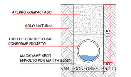
DETALHE - ASSENTAMENTO DE TUBULAÇÕES
